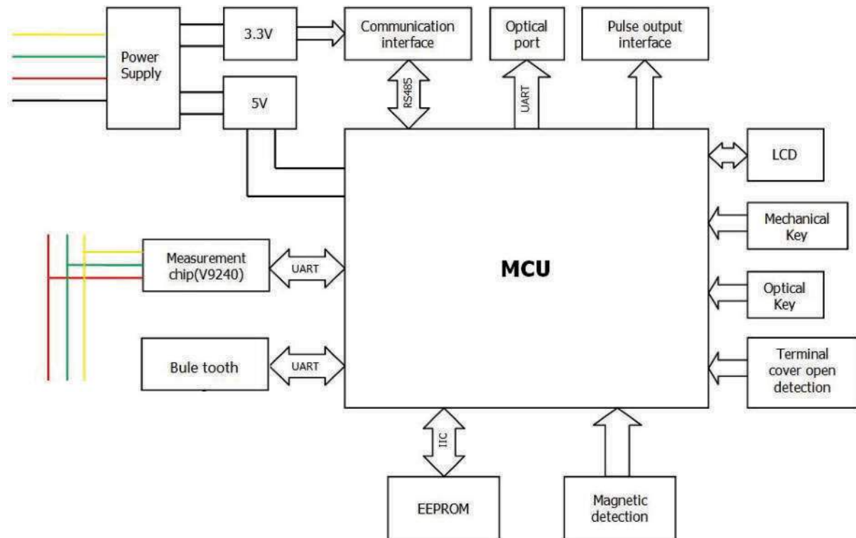
Bild 13: Blockdiagramm
