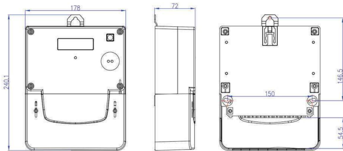
Bild 2: Abmessungen Gehäuse
