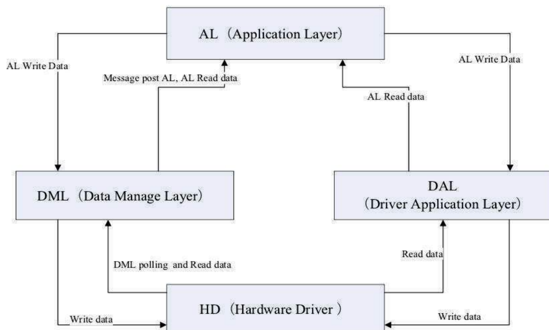
Bild 14: Firmware Struktur
