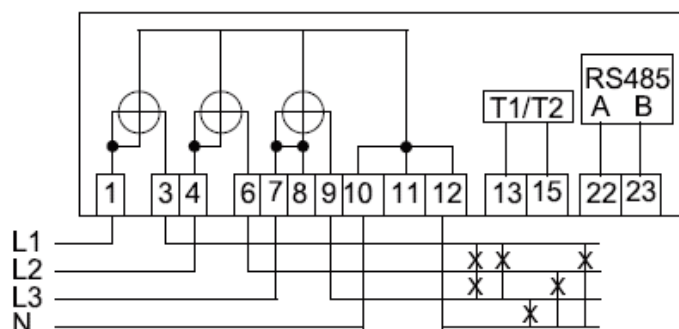
Bild 4: Schaltbild
