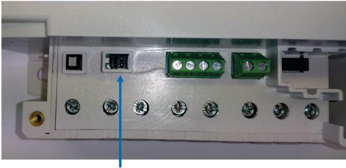
Bild 7: Hilfsspannungsanschluss
