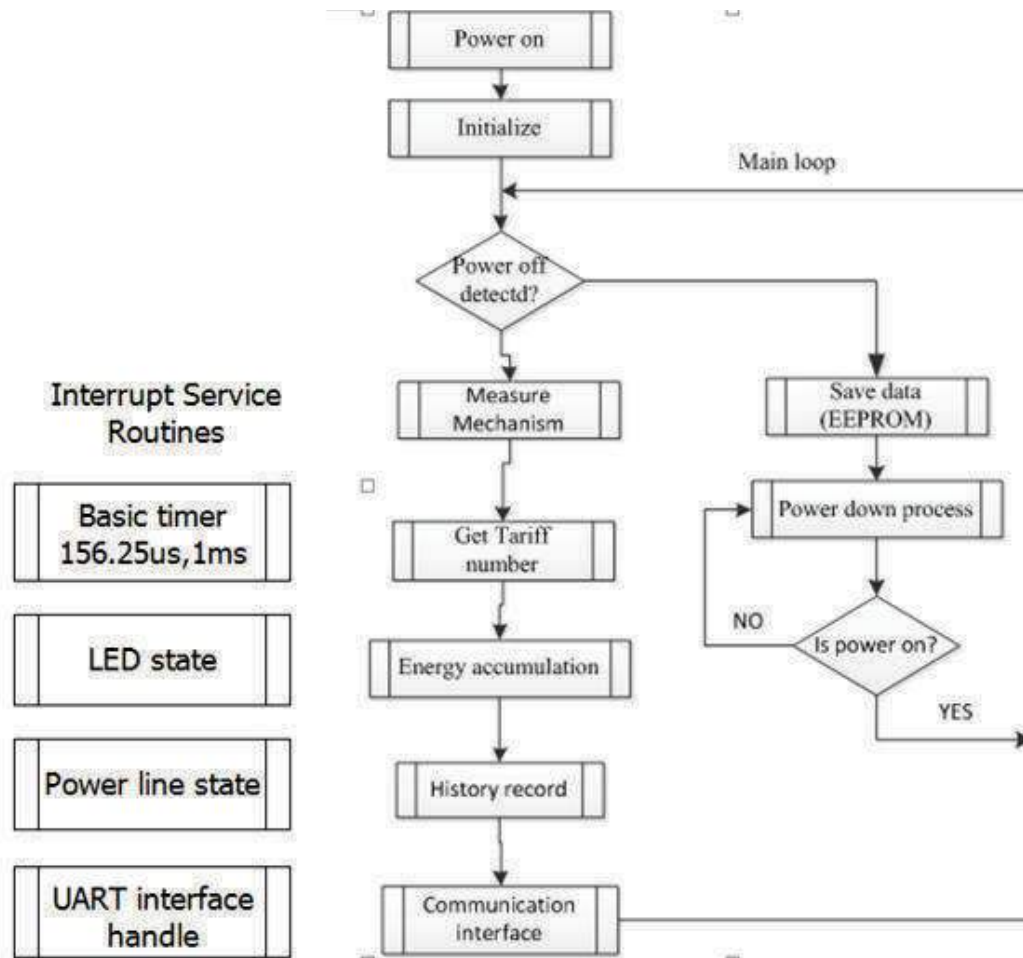
Bild 15: Firmware Flussbild
