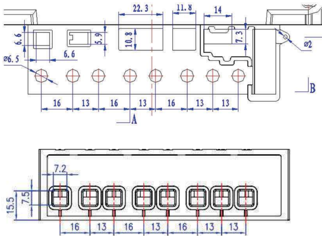
Bild 3: Klemmenblock
