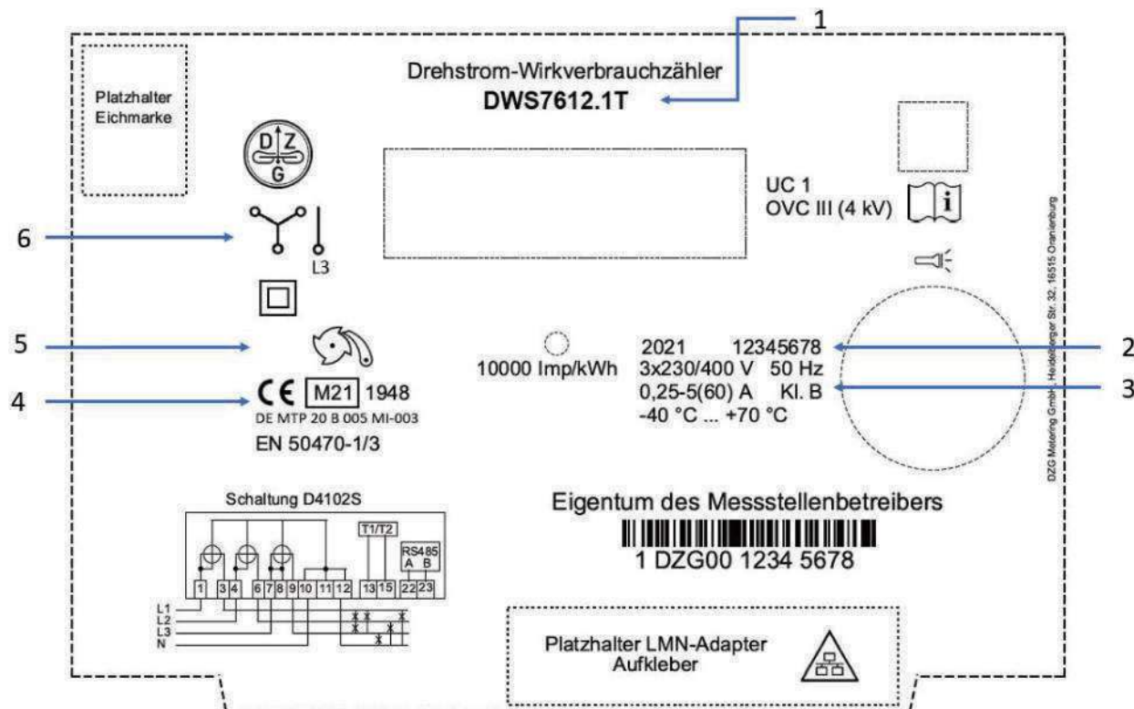
Bild 9: Leistungsschild
