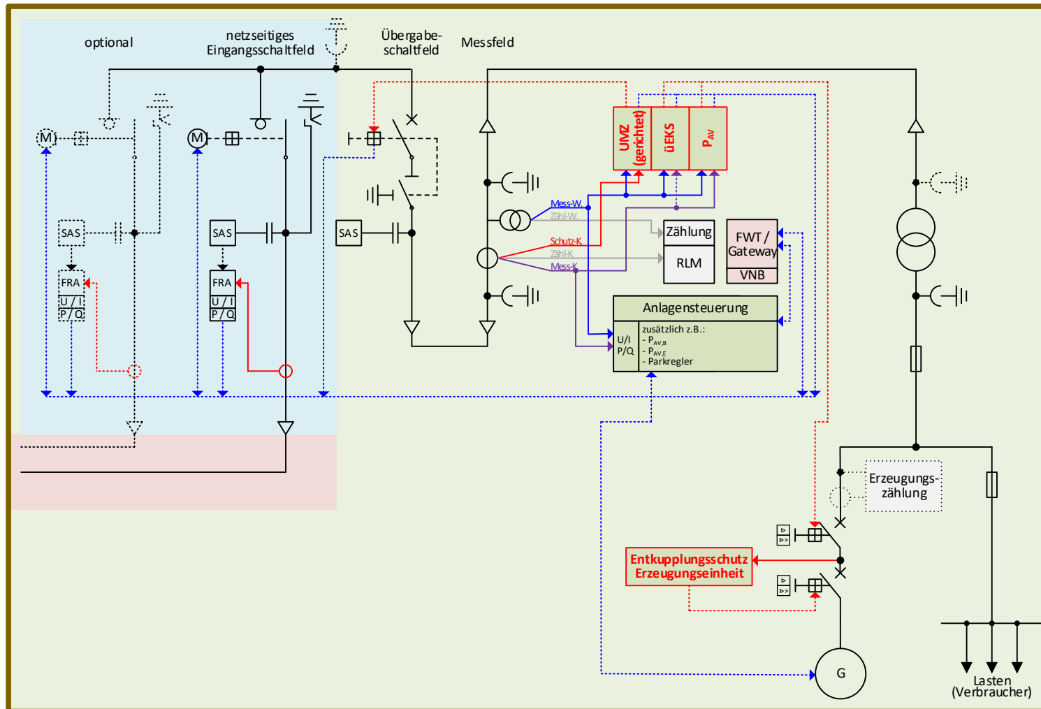
Bild D4c (K)K-TM und \Sigma P_{E_{\max}} > 500 \text{ kW} oder P_{AV,E} > 270 \text{ kW} : MS-Mischanlage – Übergabeschalter als Leistungsschalter, ein Transformator bzw. grundsätzlicher Aufbau kleiner Mischanlagen
